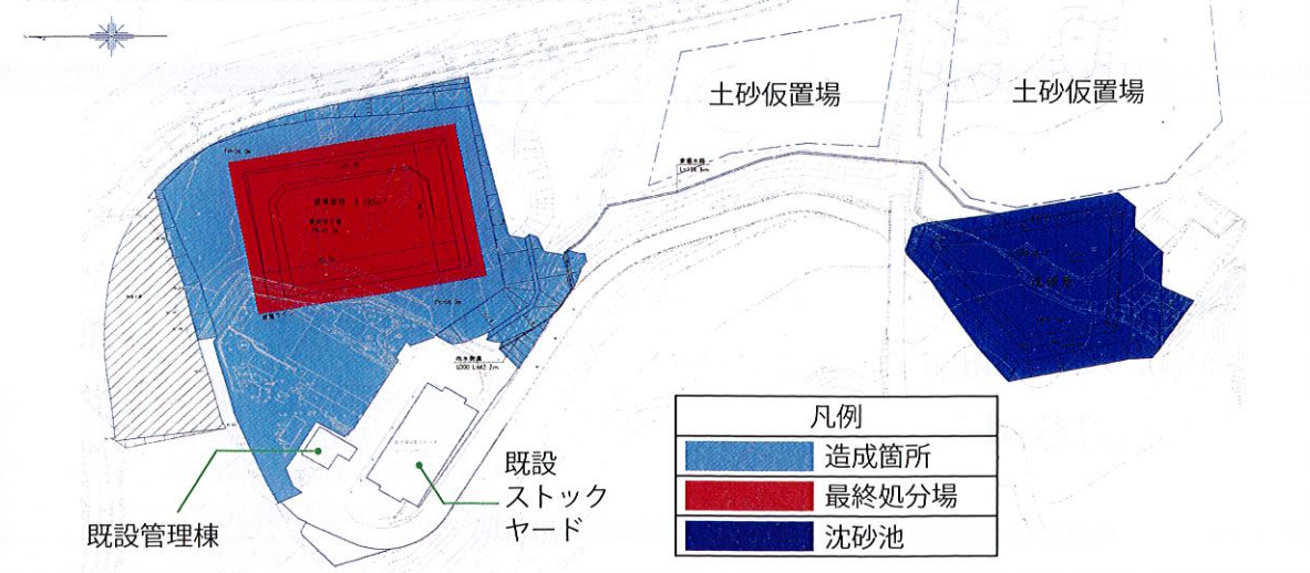
平成27年度一般廃棄物最終処分場建設実施配置図
